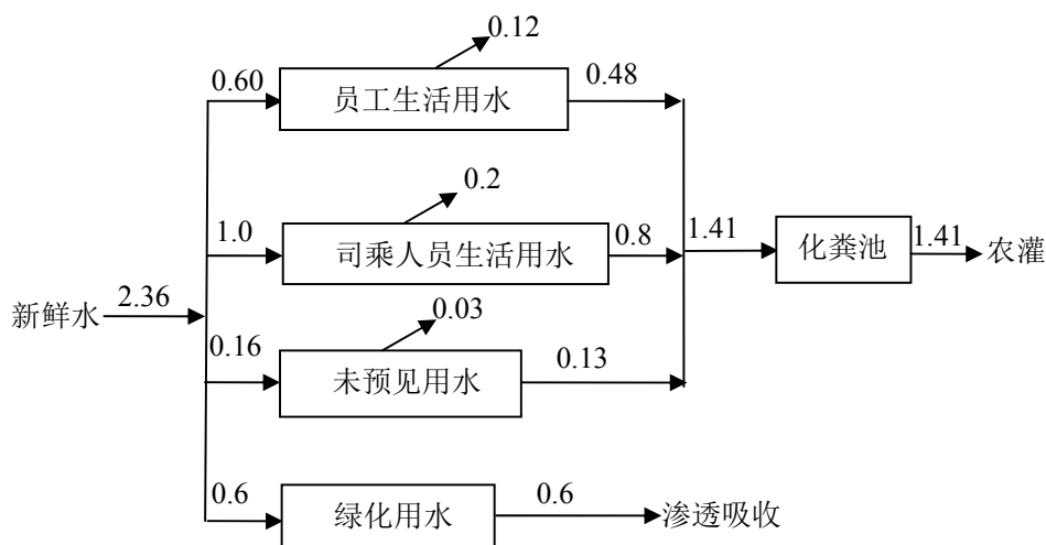
图 1-1 项目水平衡图 (单位: m 3 /d)
