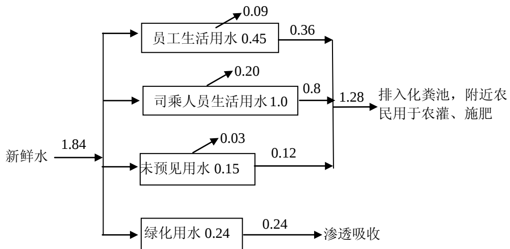
图 1-1 项目水平衡图（消耗单位：m³/d）
