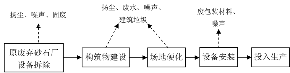
图 1：施工工艺流程及产污环节图
