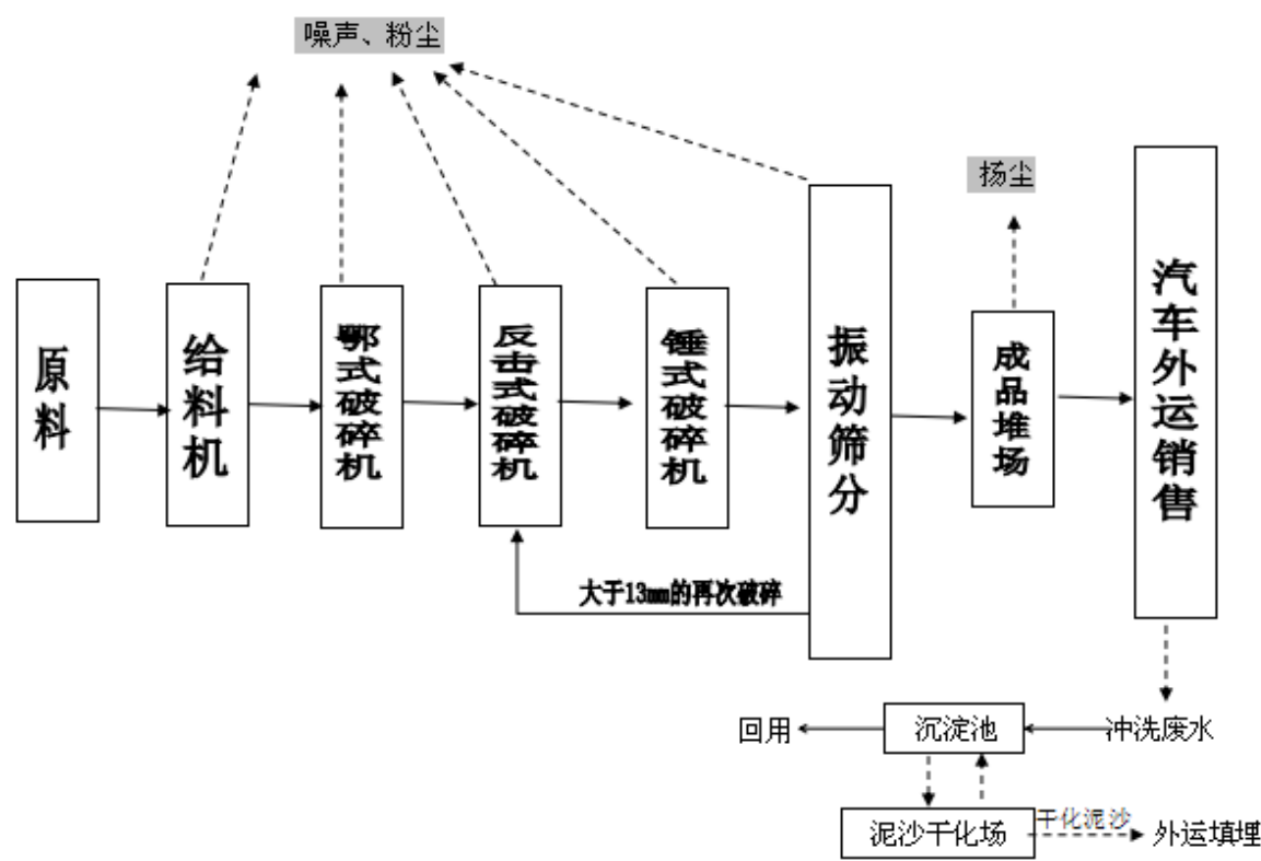
图 2：营运期工艺流程及产污环节图
